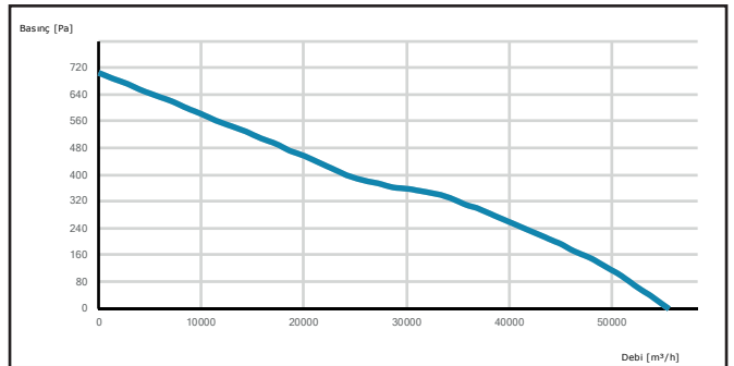
HCTAXI 1000-5-40
