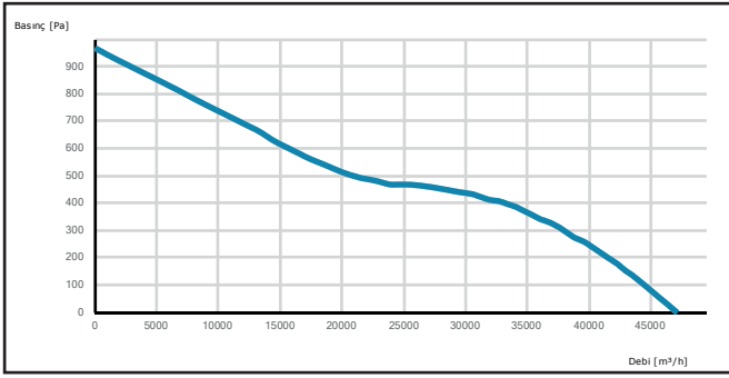
HCTAXI 900-8-40
