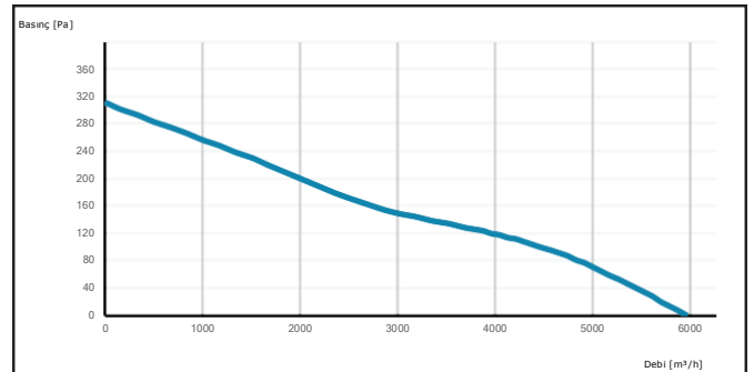
HCTAXI 500-5-25
