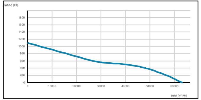
HCTAXI 1000-8-40
