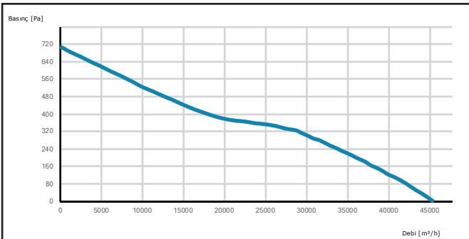
HCTAXI 900-5-40
