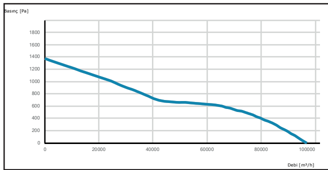
HCTAXI 1120-8-45
