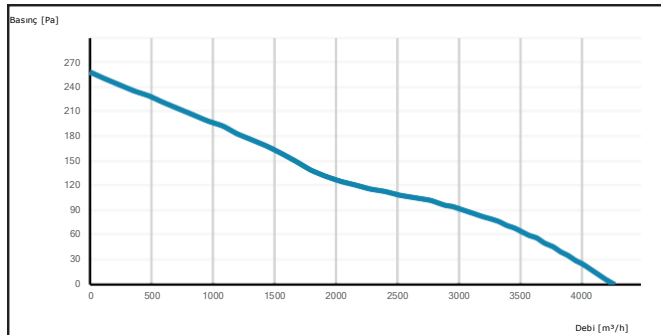
HCTAXI 450-5-25
