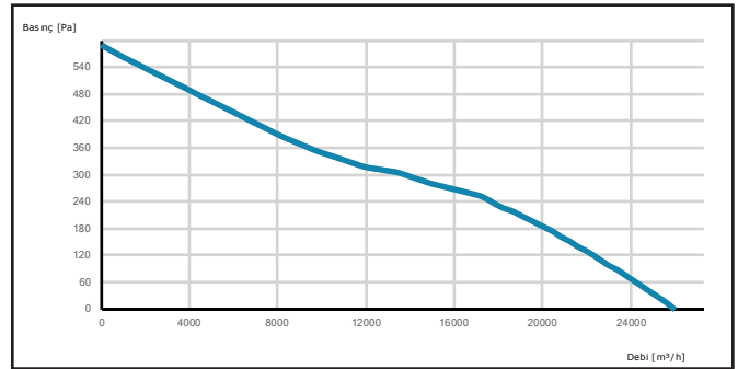
HCTAXI 800-5-30
