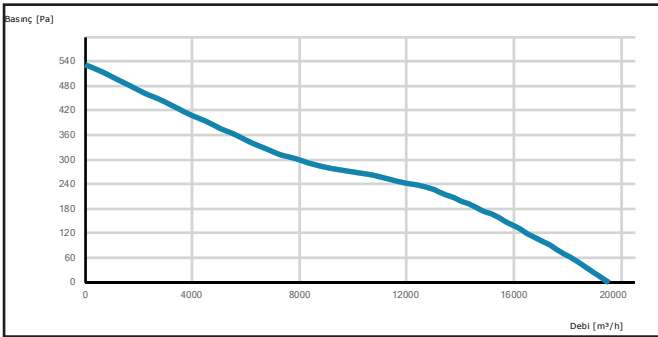
HCTAXI 710-5-30
