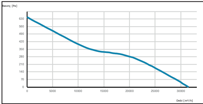
HCTAXI 800-5-35
