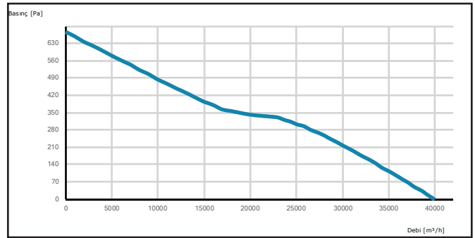
HCTAXI 900-5-35
