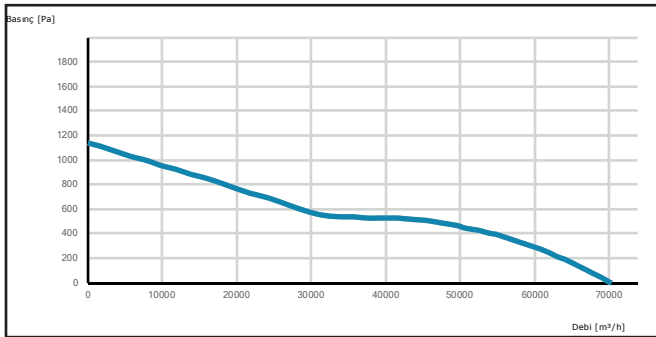
HCTAXI 1000-8-45
